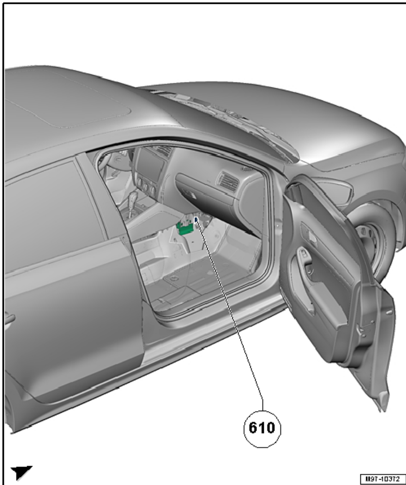
610 Точка соединения с массой (аудио) спереди под центральной консолью q момент затяжки 9 Нм
