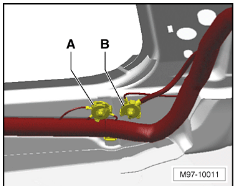
602 Точка соединения с массой в пространстве для ног в передней левой части салона -А- момент затяжки 9 Нм
